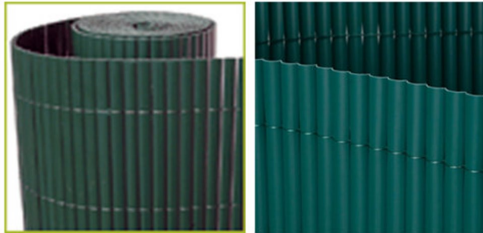
TEJIDO DE VARILLA SIMPLE CUBIERTA DE 1 SOLA CAPA COLOR VERDE 18 MM DE ANCHO LA PIEZA = 1,1 kg/m2 UNIDOS CADA 10 CM POR ALAMBRE DE NYLON
